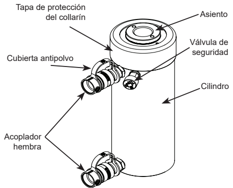
Figura 1: Componentes habituales del cilindro
